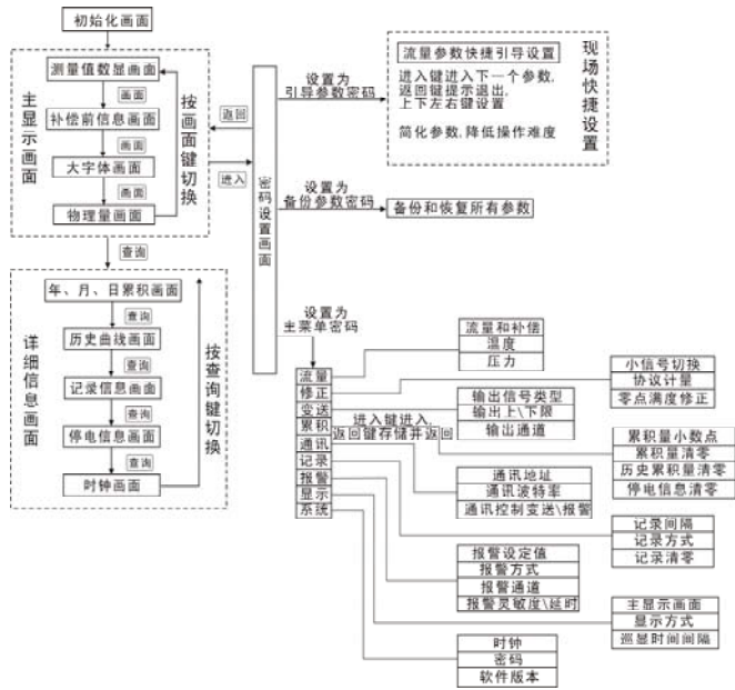
图 3 运行和操作流程图
