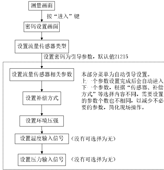
图 1 快捷操作流程图
