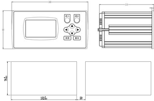
图 1 仪表外形尺寸
